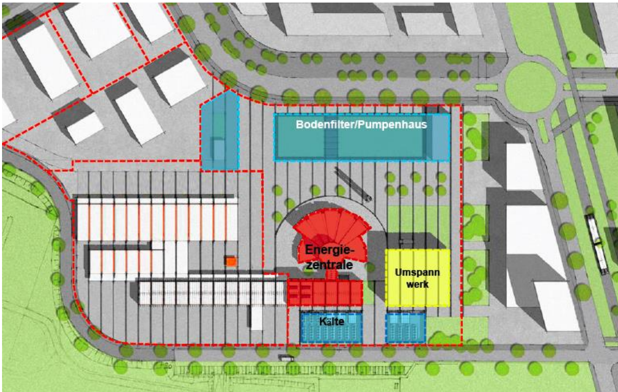
Abb. 12: Verortungsvariante der Retentionsbodenfilteranlage (Umgebung der Energiezentrale, BÜRO HAPOLD ENGINEERING/GMP ARCHITEKTEN, OKTOBER 2016)
